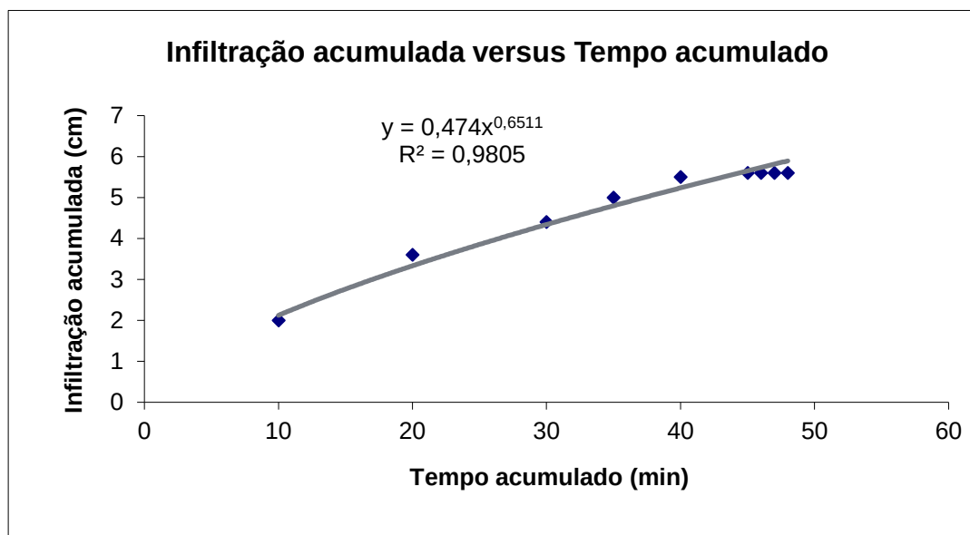
Figura 04: infiltração acumulada versus tempo acumulado
