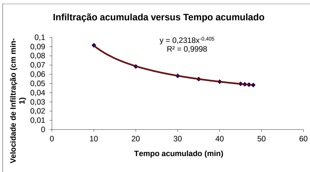
Figura 05: velocidade de infiltração versus tempo acumulado
