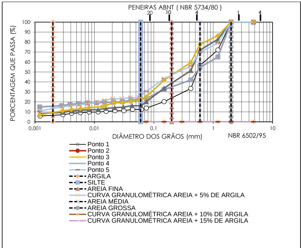
Figura 03- Curva Granulométrica
