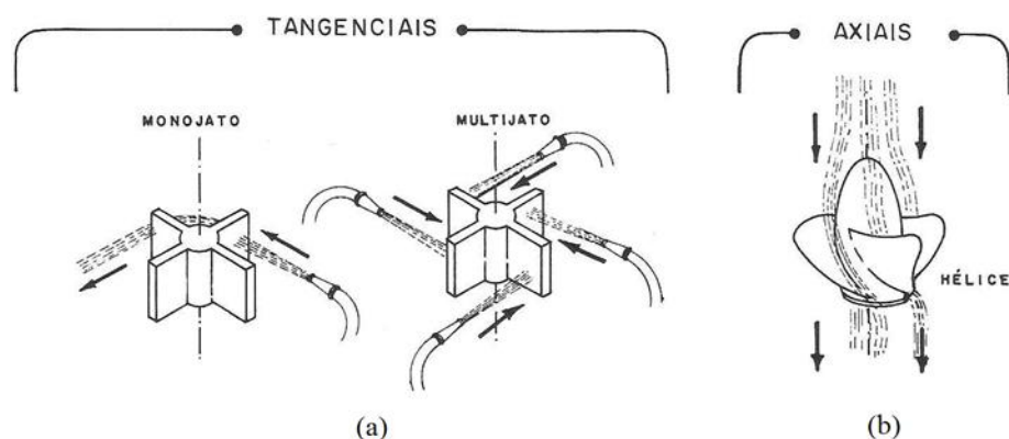
Figura 5- Hidrômetro monojato, multijato e axial
